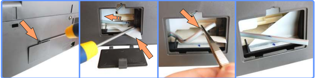
Извлечение капилляра стока CX7300
